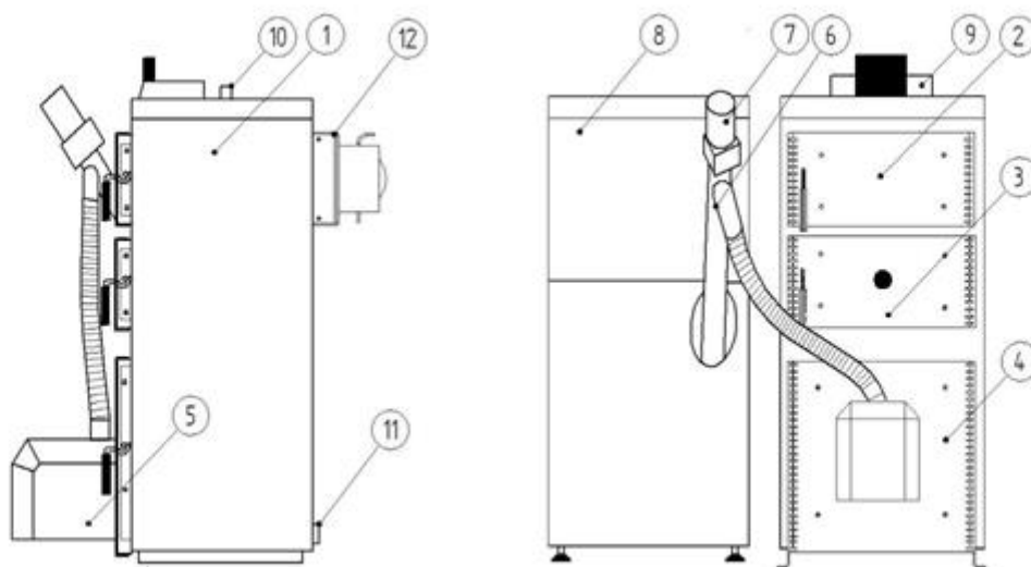
1- korpus z izolacją termiczną, 2- drzwiczki wyczystne, 3- drzwiczki obsługowe, 4- drzwiczki popielnikowe, 5-palnik, 6- podajnik paliwa, 7- motoreduktor, 8-zbiornik paliwa, 9-regulator mikroprocesorowy, 10- króciec zasilania, 11- króciec powrotu, 12-czopuch.
