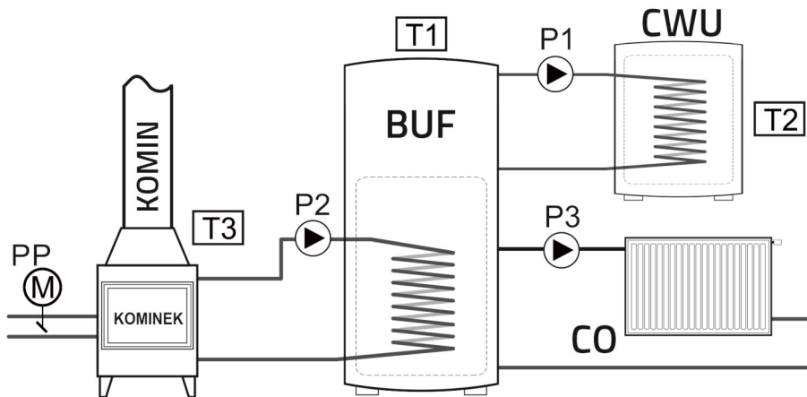
Rys.1a Podstawowy układ pracy regulatora (CWU za BUF). Parametr „<93> CWU przed BUF”=WYL.
