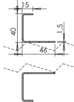
PRZEKRÓJ A-A SKALA 1 : 3
